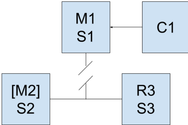
Рис. 575 — Разделение сети
